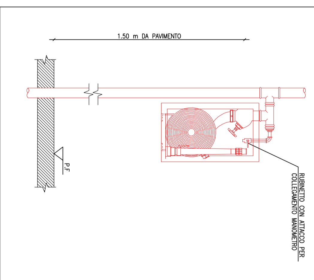
TIPICO IDRANTE A MURO UNI45 (FUORI SCALA)
